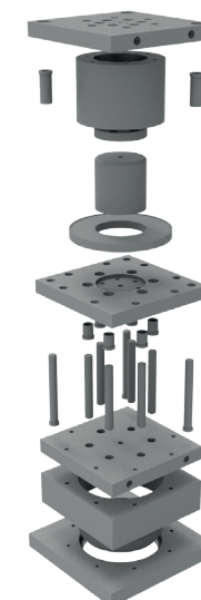
Штамп вытяжной
