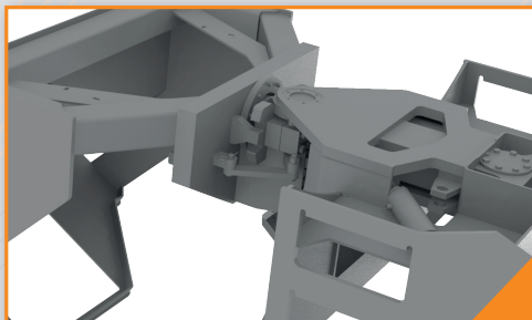
Шарнир с крабовым ходом для тандемного катка
