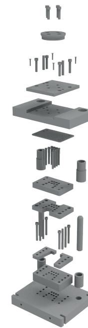
Штамп пробивной
