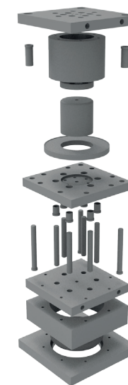
Штамп вытяжной
