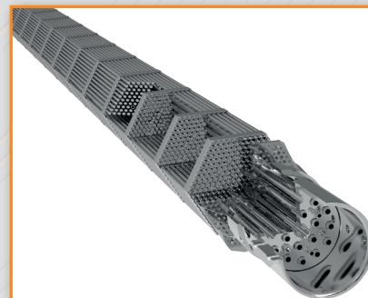
Тепловыделяющий элемент
