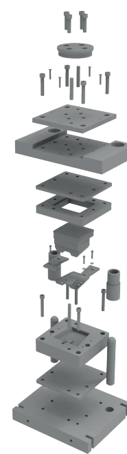
Штамп формовочный
