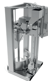
Дегазатор алюминиевых расплавов
